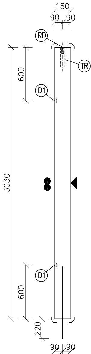
ŘEZ A-A
